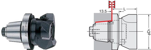
クイック型プロカット(2面拘束型)
