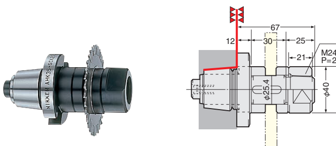
クイック型サイドカッターアーバ(2面拘束型)
