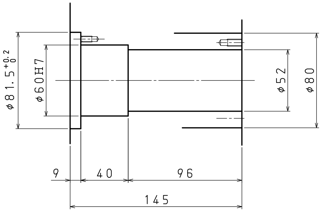
DETAIL OF CENTER BORE (S=1/2) センター穴詳細 (S=1/2)
